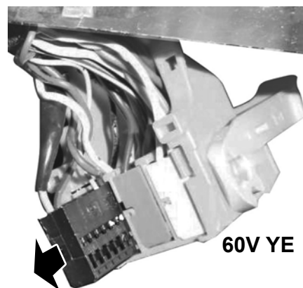
BSI - Conn EH2 - 60V YE
