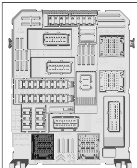
BSI - Conn EH2 - 60V YE
