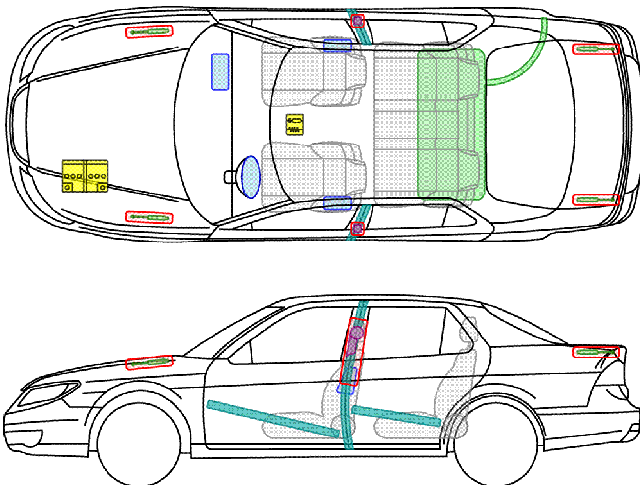
Turvatyyny
